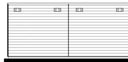
ACHTERAANZICHT
