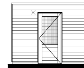
ZIJAANZICHT LINKS
