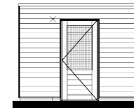
ZIJAANZICHT LINKS
