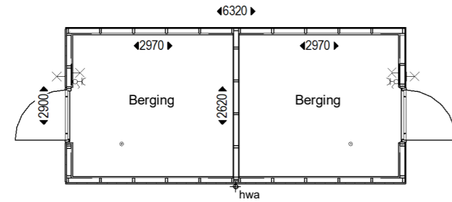
PLATTEGROND
