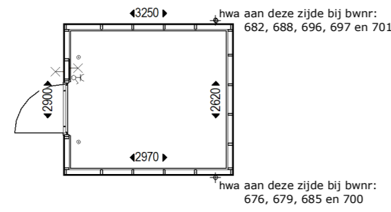
PLATTEGROND
