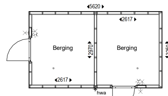
PLATTEGROND
