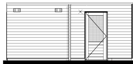
VOORAANZICHT
